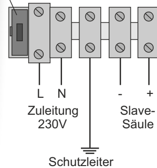
Sicherung 230V Zuleitung
