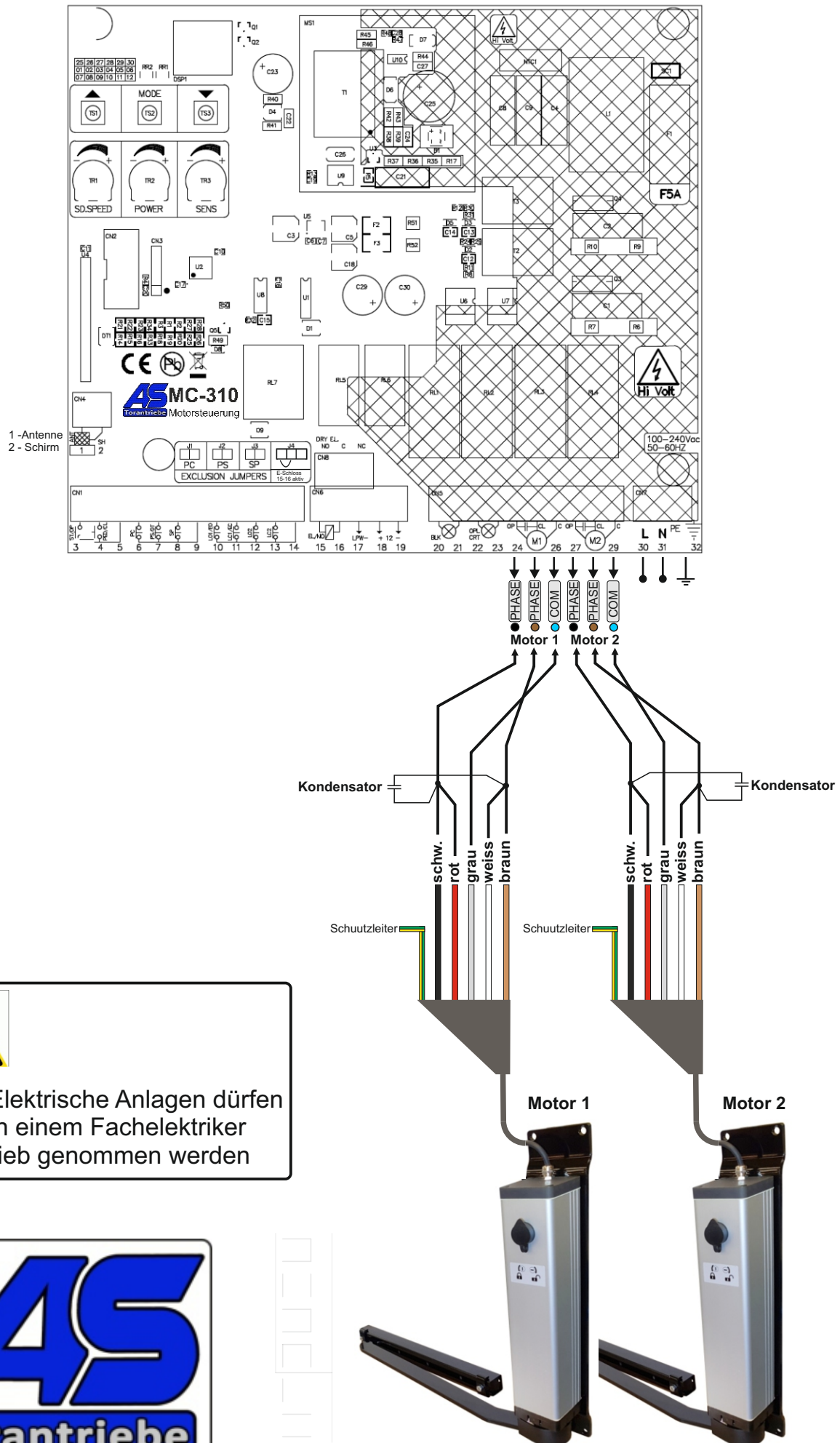
Motorsteuerung MC-310
