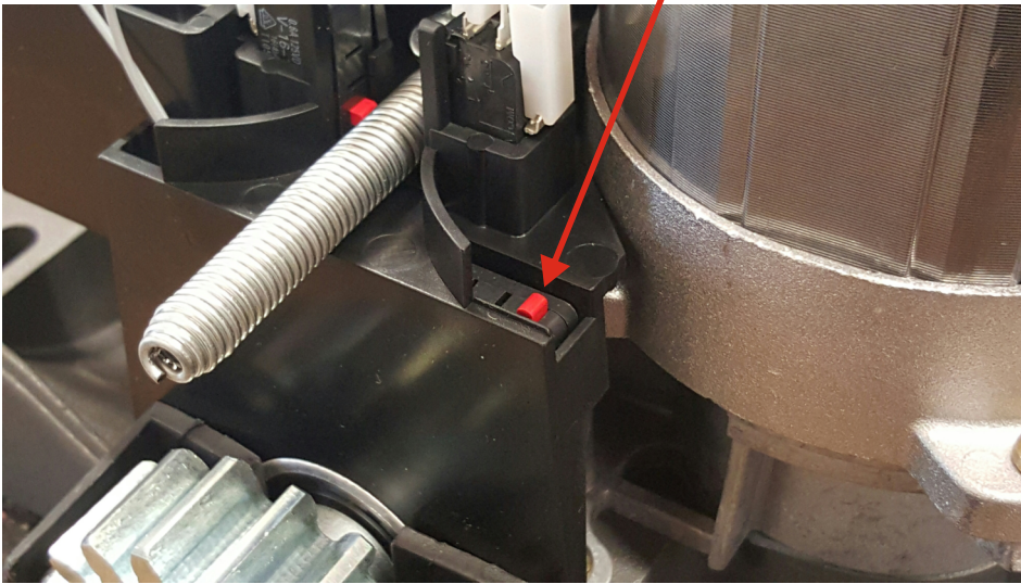
Endschalter - Haube
