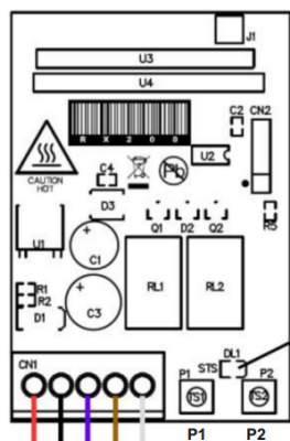
Empfänger RX-200
