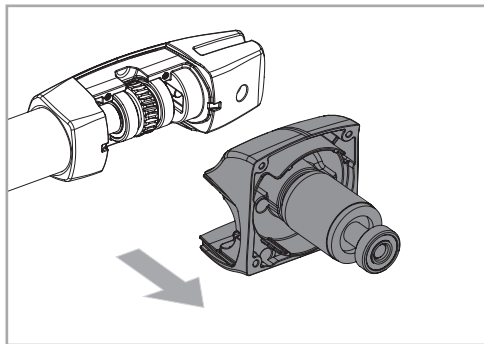
04 • Entfernen Sie den mittleren Teil.
