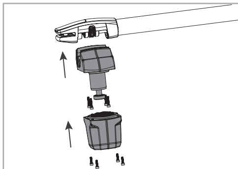
06 • Befestigen Sie den Antrieb in dem Sie die Automatisierungskomponenten anschrauben.
